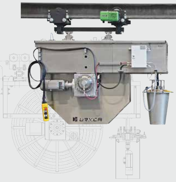
Kombination aus manueller Positionier- vorrichtung mit automatischem Haspelsystem und autarker Steuereinheit
